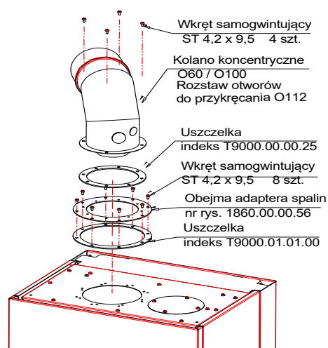
Układ koncentryczny
