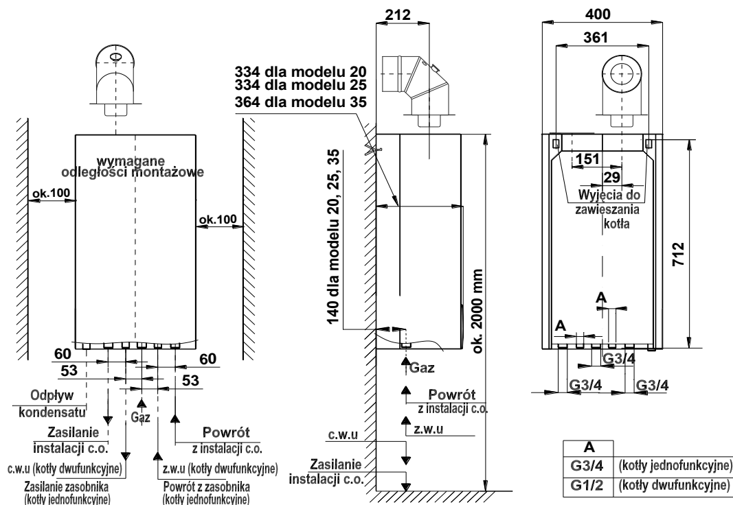
Rys. 3.3.1 Wymiary instalacyjne kotłów ECOCONDENS GOLD
