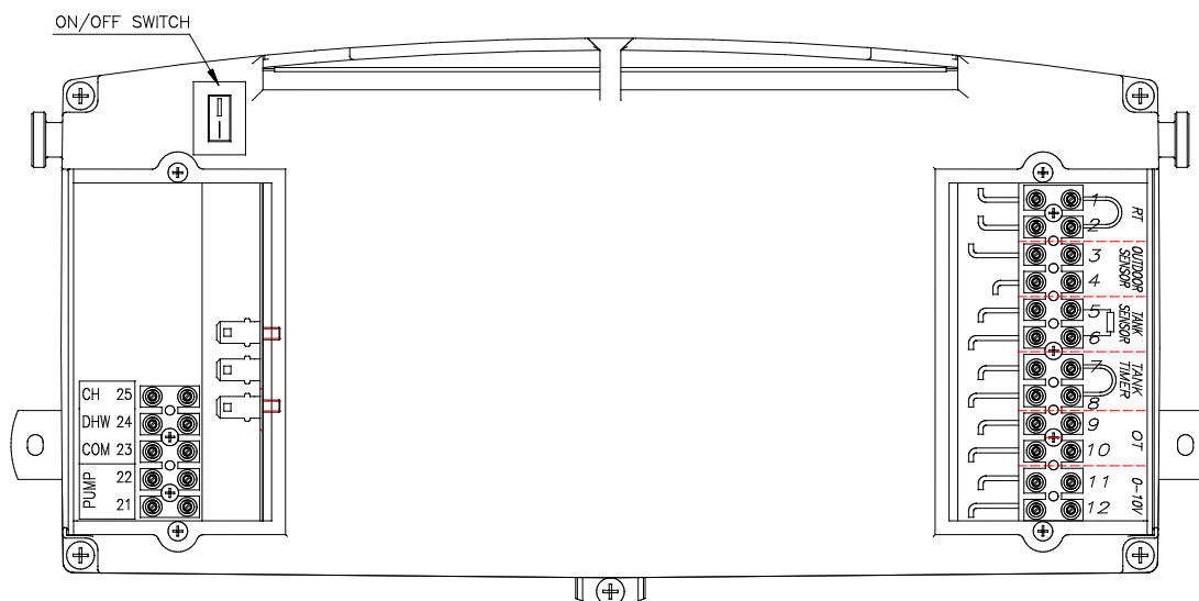
Rys.3.9.1 Zaciski elektryczne sterownika kotłów dwu-funkcyjnych
