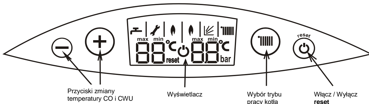
Rys. 5.2.1. Panel sterowania
