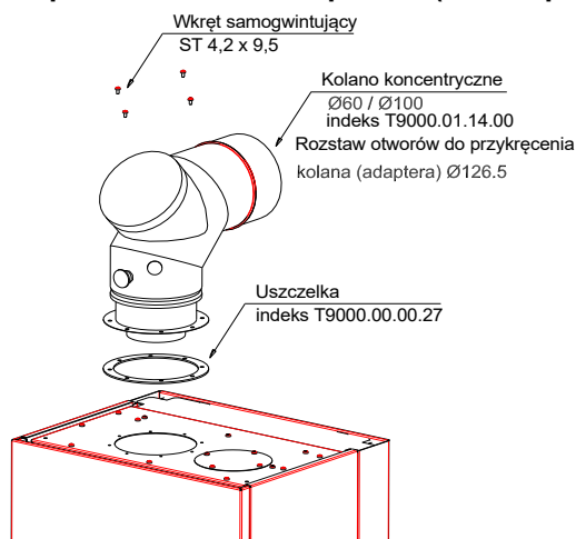
Układ koncentryczny
