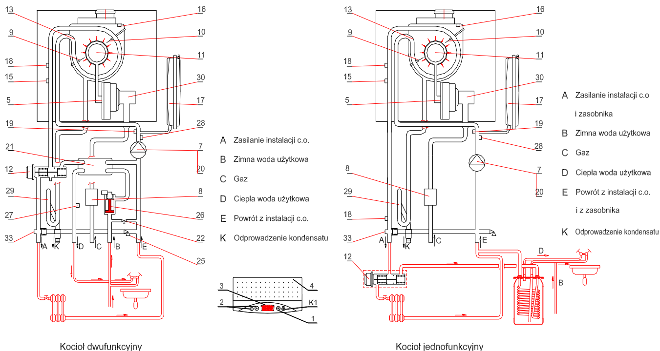
Rys.2.2.1.3. Schemat ideowy działania kotła
