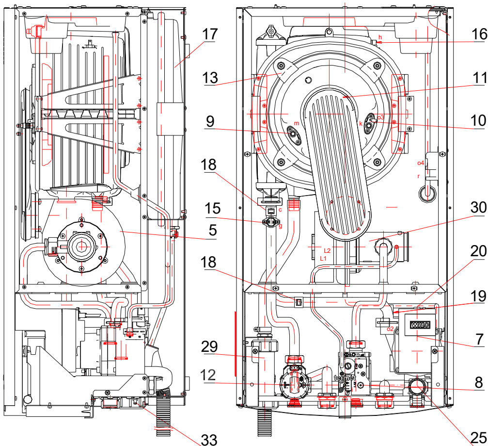
Rys.2.2.1.2. Rozłożenie elementów w kotle ECOCONDENS GOLD jednofunkcyjnym
