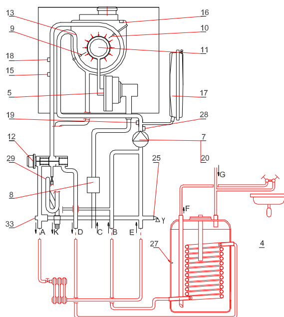
Rys.2.2.1.2. Schemat ideowy
