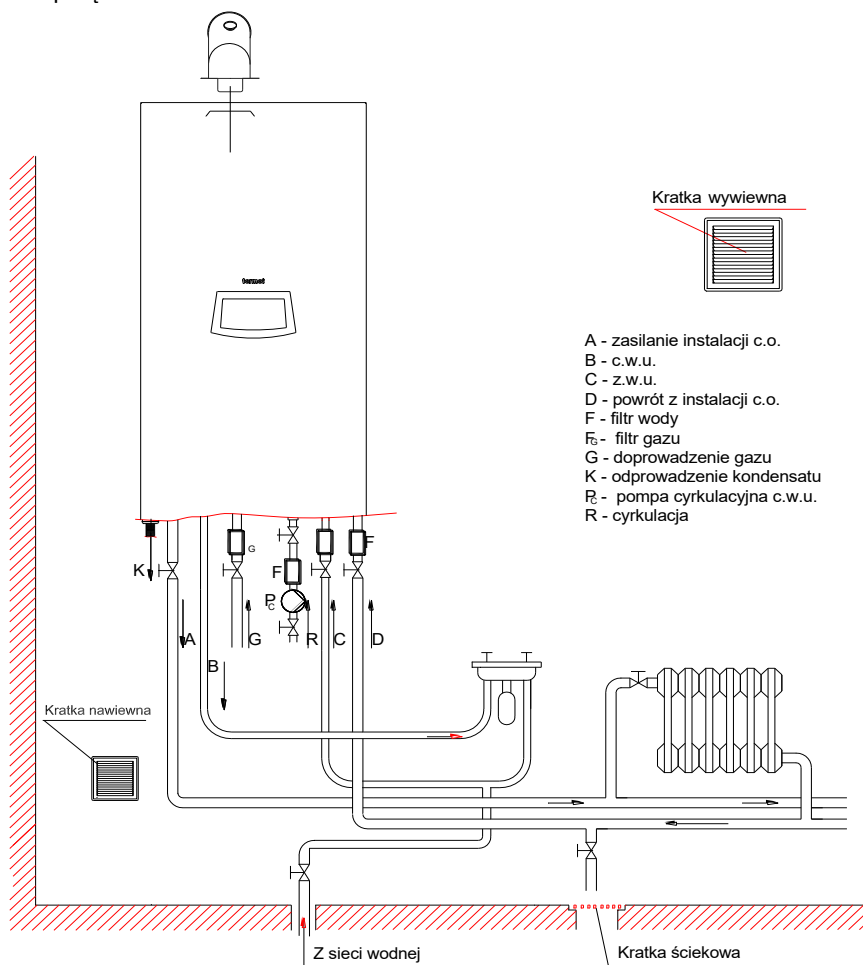
Rys.3.5.1 Wymagania instalacyjne kotłów
