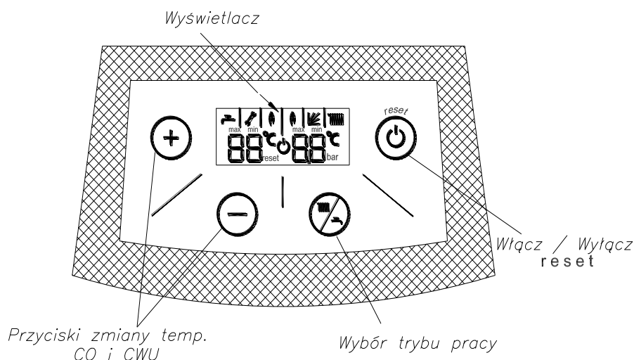
Rys. 5.2.1. Panel sterowania
