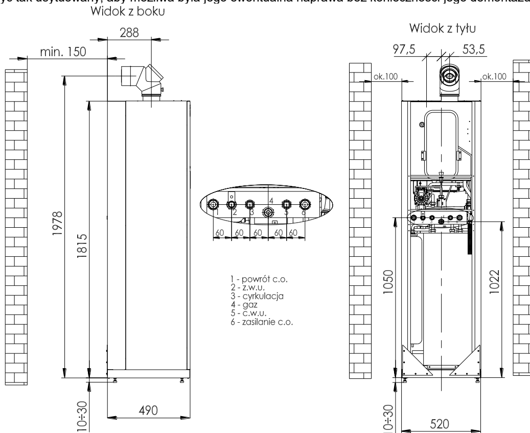
Rys. 3.3.1 Wymiary instalacyjne kotłów typ ECOCONDENS SOLID
