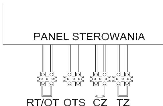
Rys.3.9.1 Płytki sterownika
