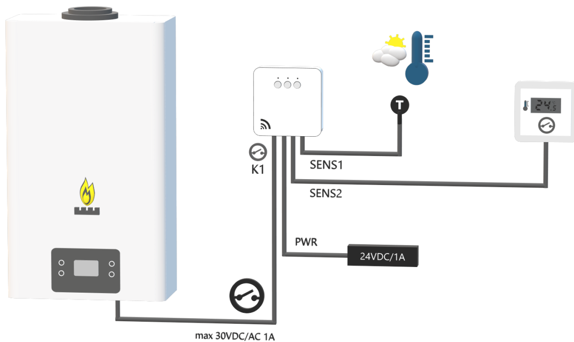
Rys 14. Konfiguracja z pobudzeniem grzania wyzwalanym przez tradycyjny (stykowy) regulator temperatury
