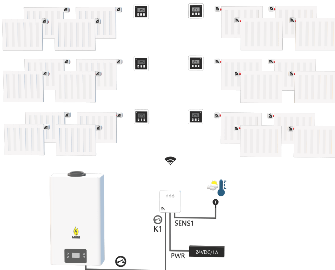
Rys 12. Konfiguracja z regulatorami stref grzewczych.
