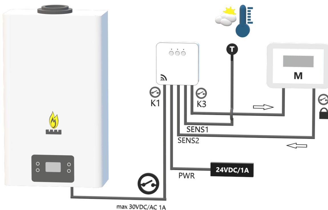
Rys 15. Konfiguracja z managerem źródeł ciepła.
