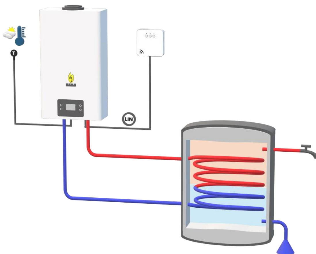
Rys 10. Konfiguracja z zasobnikiem wody użytkowej (podłączenie interfejsem LIN).
