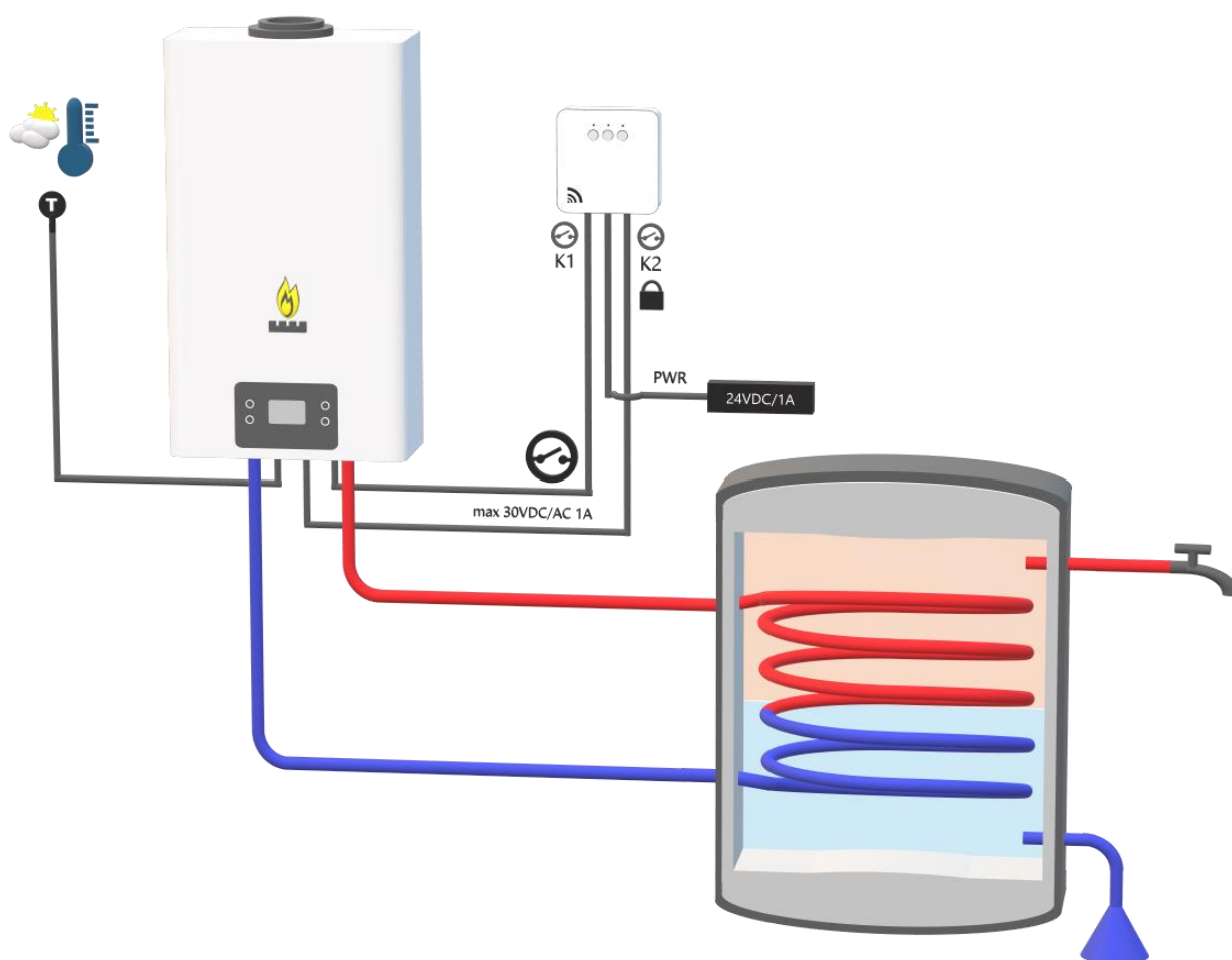
Rys 16. Konfiguracja z zasobnikiem wody użytkowej (blokada pracy na zasobnik stykiem sterującym K2).
